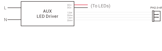
Sensor Wiring
