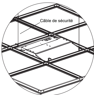
Figure 3: Utiliser des câbles de soutien pour fixer le luminaire.
