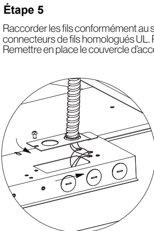
Figure 4: Réalisation des raccordements électriques.
