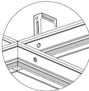
Figure 2: Installation du luminaire dans le système de plafond en treillis en T.
