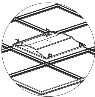
Figure 1: Pliage des attaches de grille.
