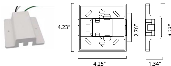
Connecteur d'alimentation à 3 fils
